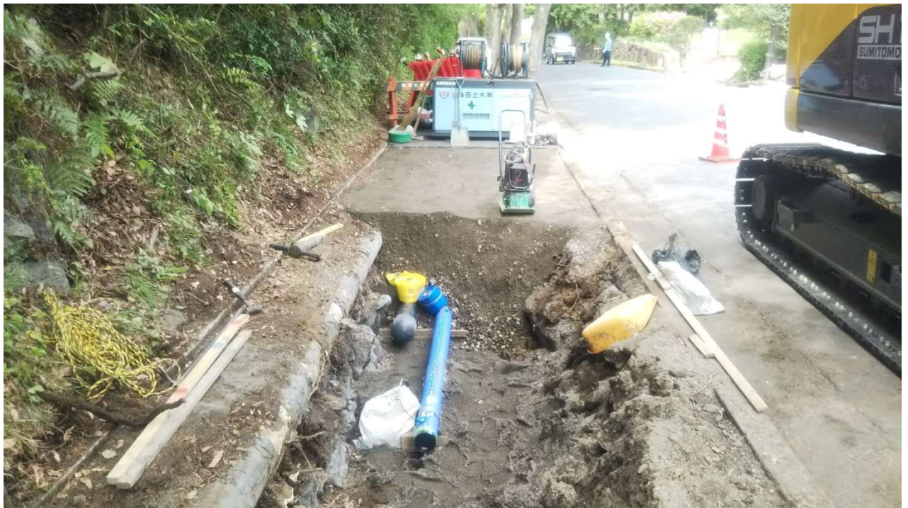
けやき通り汚水管・温泉管 更新工事状況 (けやき通り)
